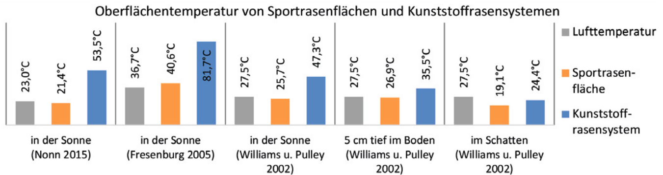
Oberflächentemperatur in Grad Celsius (°C) von Sportrasenflächen und Kunststoffrasensystemen
