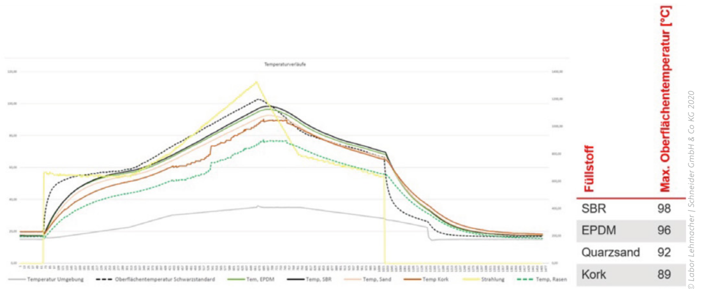
Messdaten zum Temperaturverlauf an einem simulierten Tag
